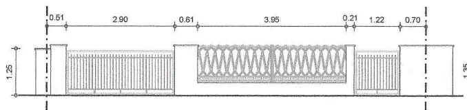
PROSPETTO RECINZIONE FRONTE STRADA
