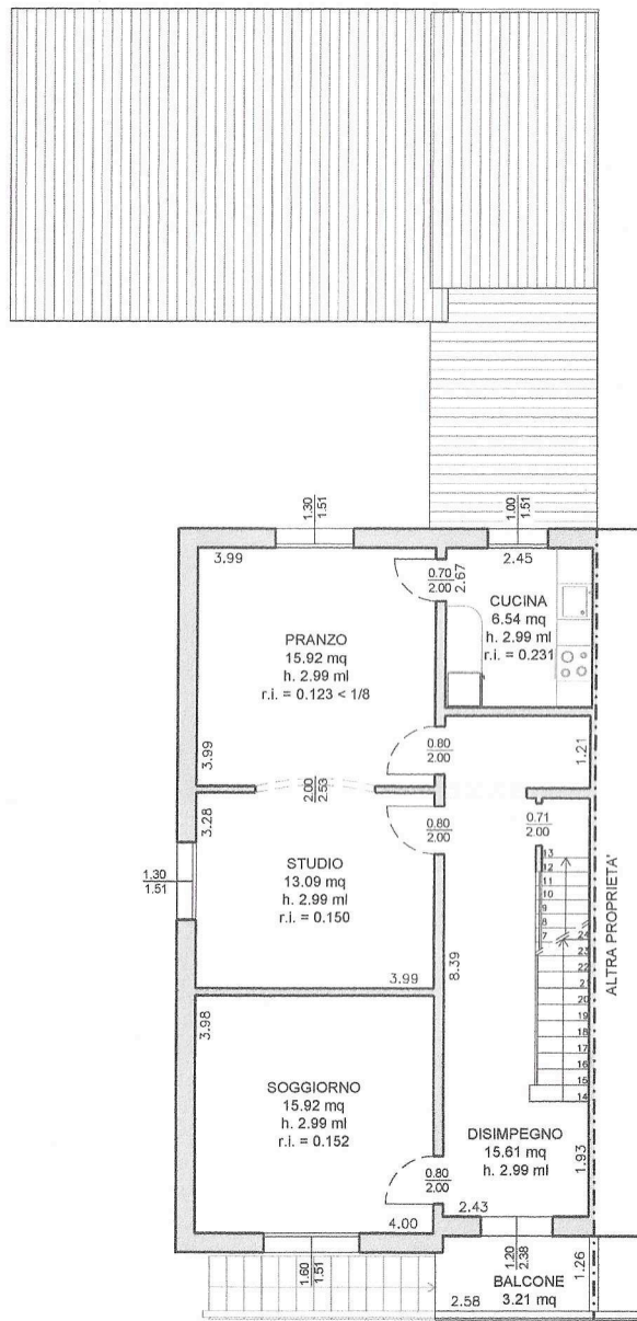
PIANTA PIANO PRIMO
